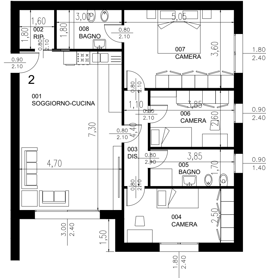
PIANTA APPARTAMENTO N.2
